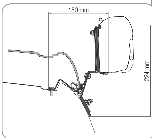
FIAMMA F45s
